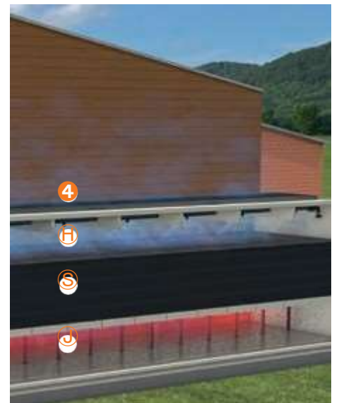
フィルターパッケージを通り排気ガスが上に流れます
