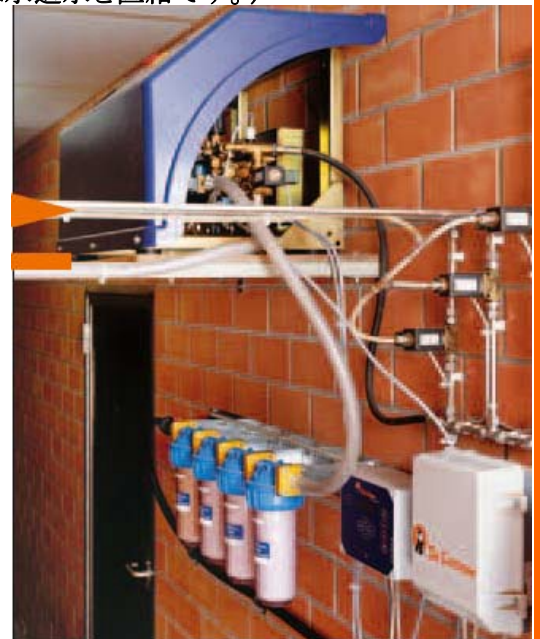
ポンプユニット周辺設置例
