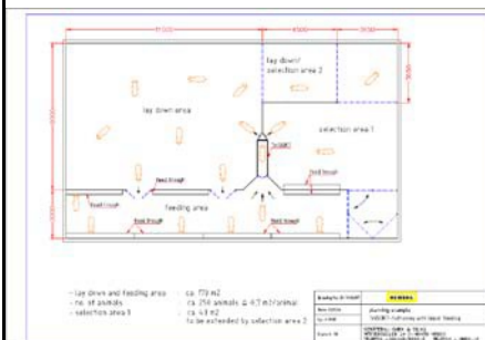
(リキッドフィーディング時の推奨レイアウト)
