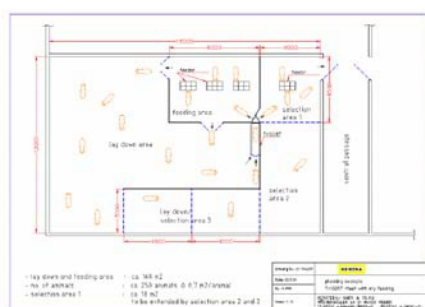
(ドライフィーディング時の推奨レイアウト)
